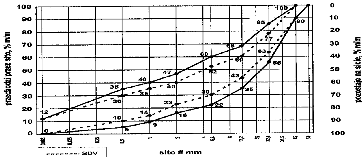
Rys. 9. Mieszanka niezwiązana 0/45 do warstw podbudowy pomocniczej
