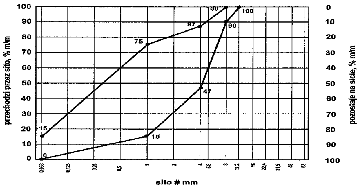
Rys. 1. Mieszanka kruszyw 0/8 do górnej warstwy ulepszonego podłoża
