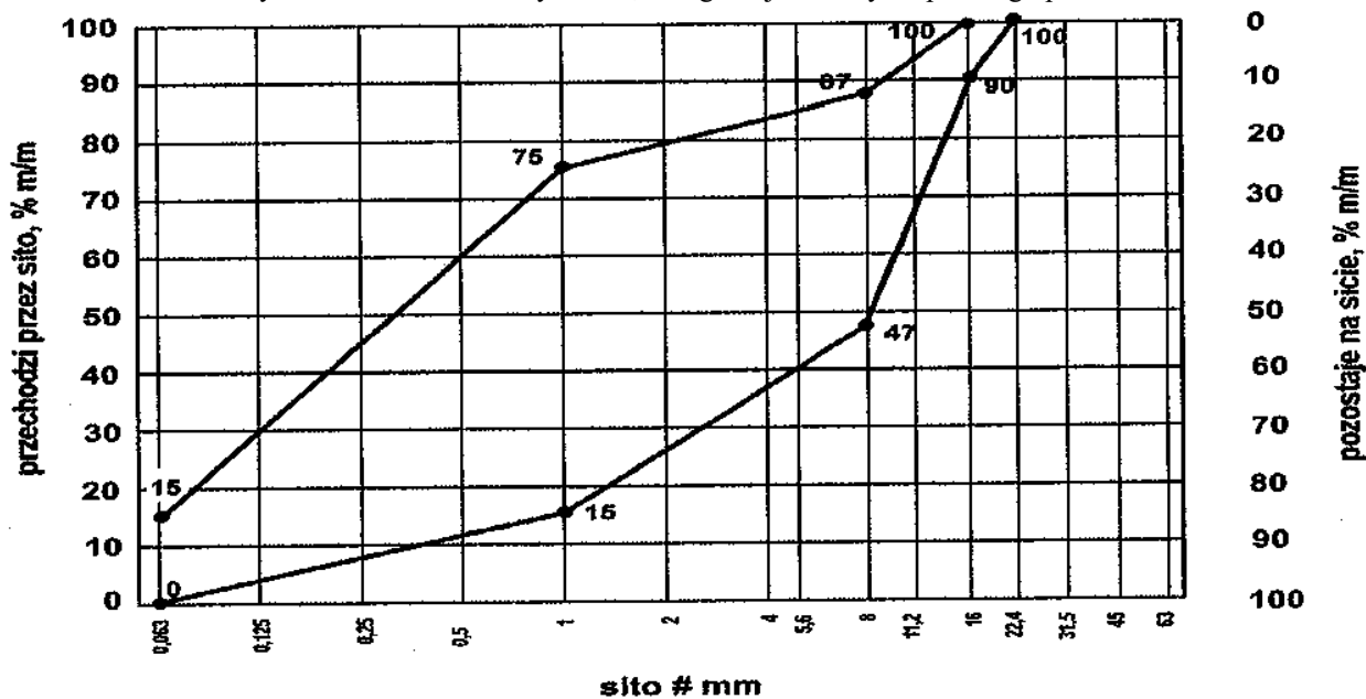
Rys. 3. Mieszanka kruszyw 0/16 do górnej warstwy ulepszonego podłoża
