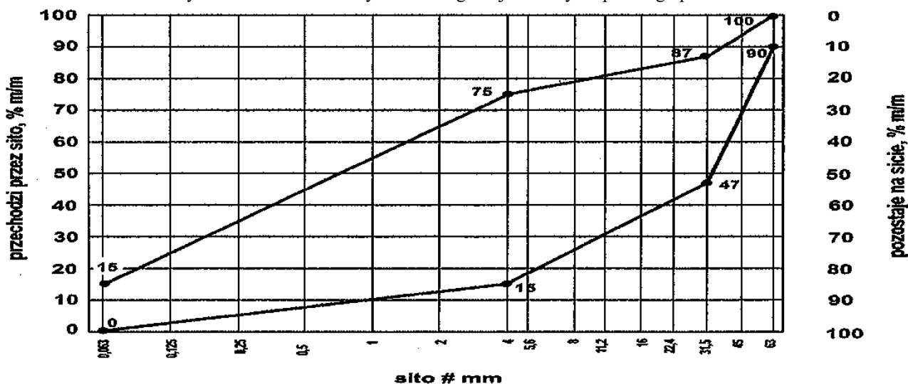
Rys. 7. Mieszanka kruszywa 0/63 do górnej warstwy ulepszonego podłoża
