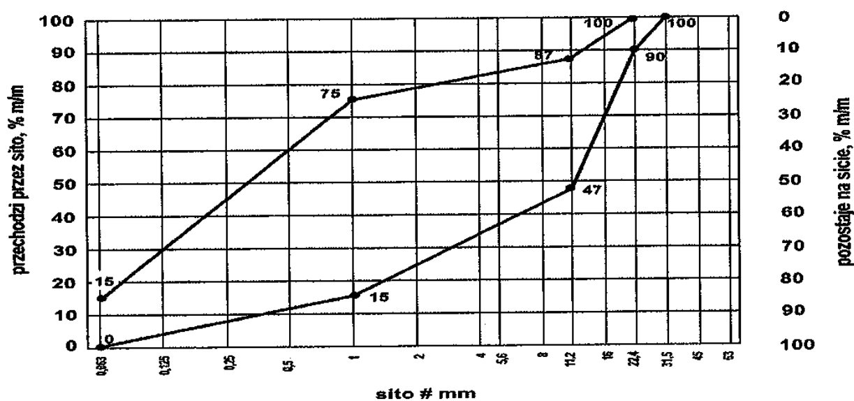
Rys. 4. Mieszanka kruszyw 0/22,4 do górnej warstwy ulepszonego podłoża
