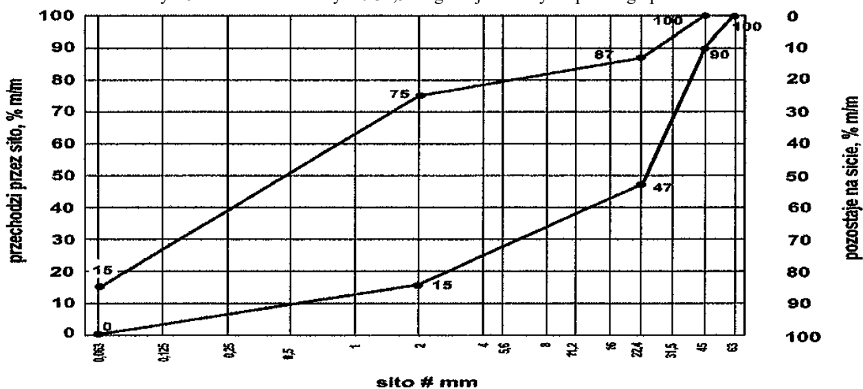
Rys. 6. Mieszanka kruszywa 0/45 do górnej warstwy ulepszonego podłoża
