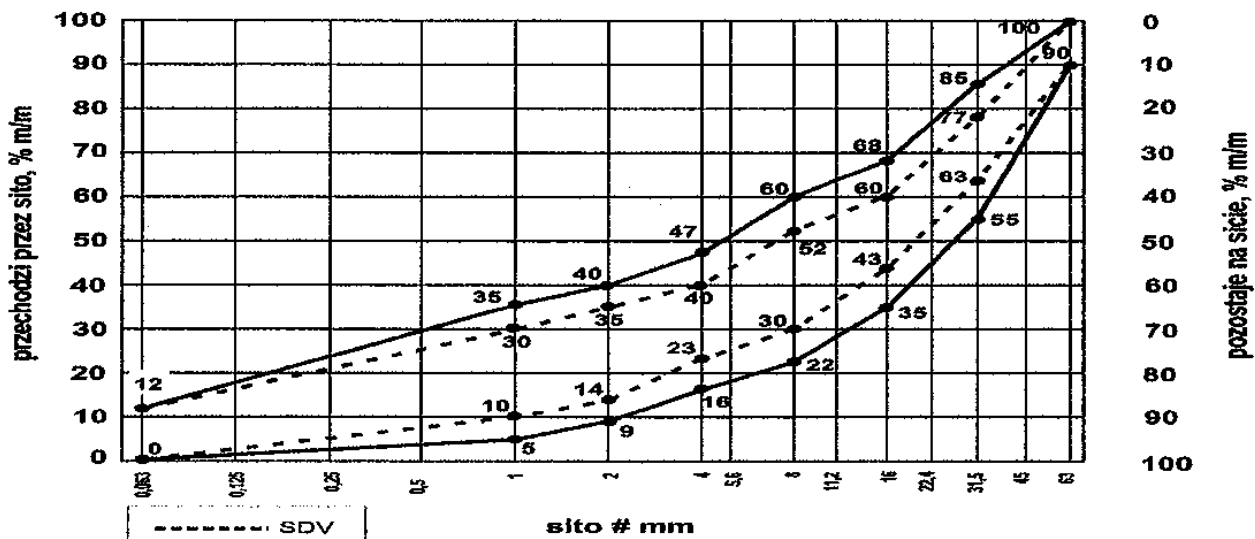
Rys. 10. Mieszanka niezwiązana 0/63 do warstw podbudowy pomocniczej
