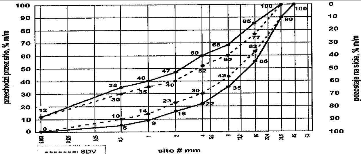
Rys. 8. Mieszanka niezwiązana 0/31,5 do warstw podbudowy pomocniczej
