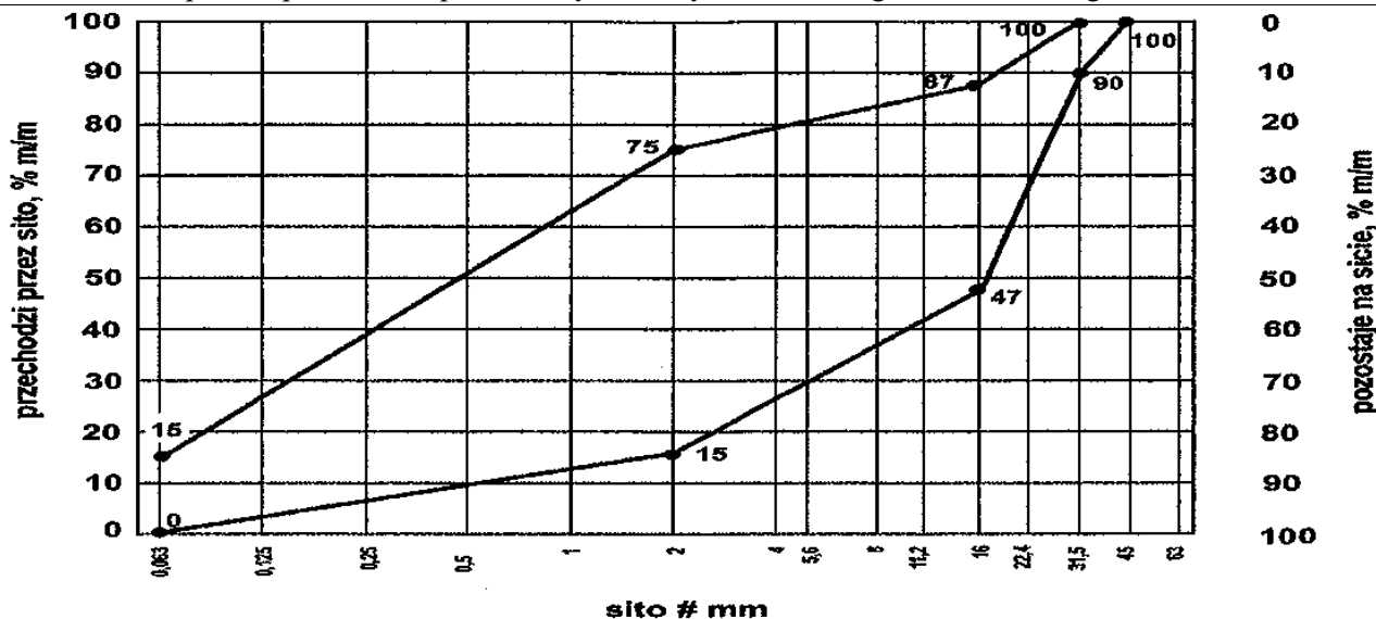
Rys. 5. Mieszanka kruszywa 0/31,5 do górnej warstwy ulepszonego podłoża
