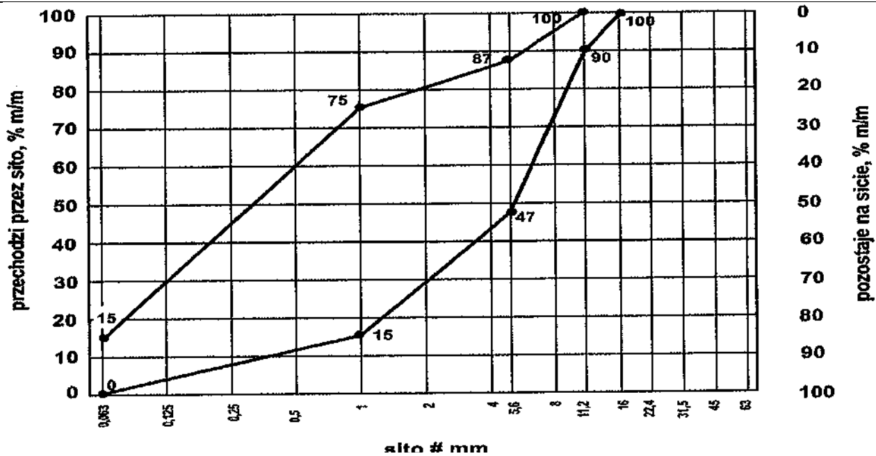
Rys. 2. Mieszanka kruszyw 0/11,2 do górnej warstwy ulepszonego podłoża
