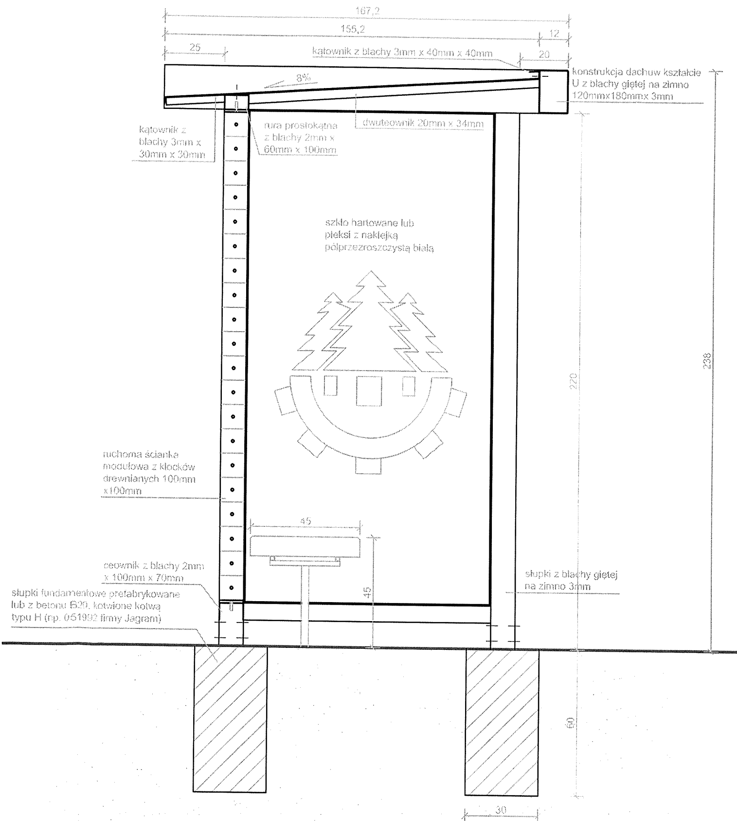
przekrój A-A średniej wiaty
