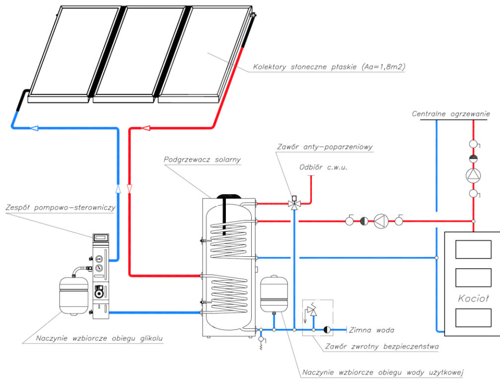
Schemat ideowy instalacji solarnej dla potrzeb c.w.u. z kotłem na paliwo stałe
