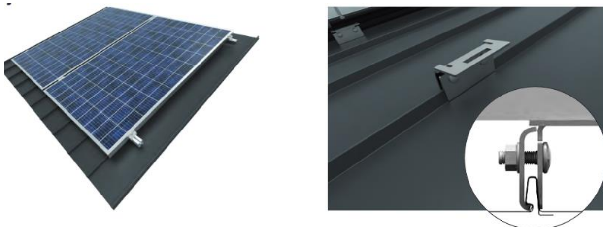
Rys. 1 Widok systemowego mocowania do dachów skośnych pokrytych blachą na rąbek.
