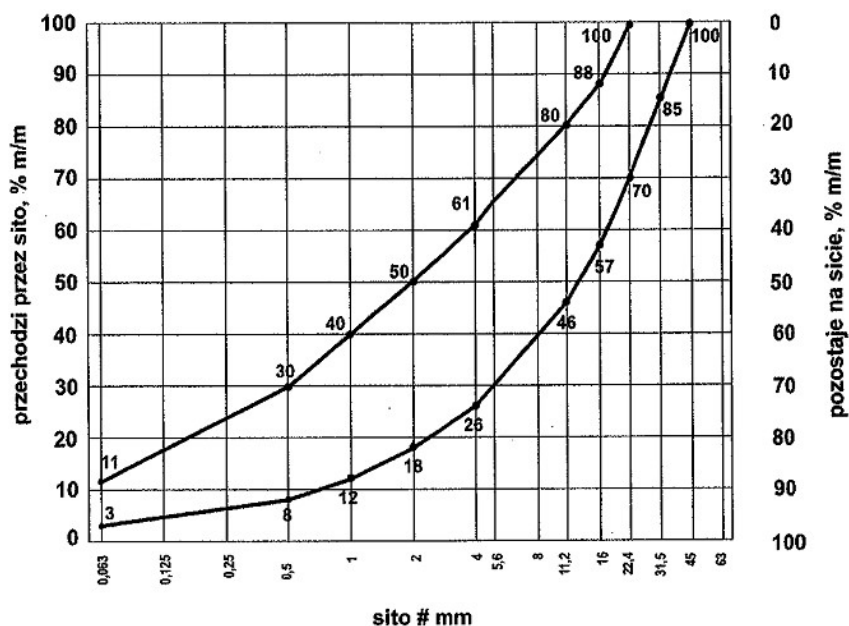
Rysunek 1 Mieszanka niezwiązana 0/31,5 do warstw ulepszanego podłoża
